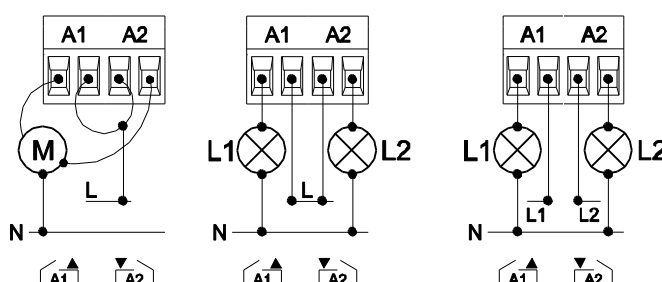
Рисунок 2: Примеры подключения: (слева направо): канал А как канал жалюзи и индивидуальные выходы канала А с одинаковыми и разными фазами.
