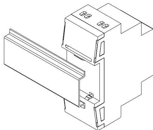
Рисунок 3: Установка MINiBOX 20 на DIN рейку
