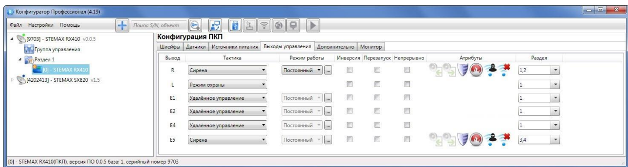
Рисунок 7.8 – Вкладка Выходы управления для ППК STEMAX RX410
