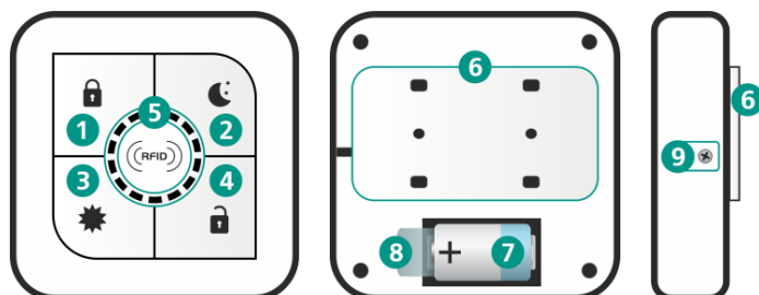
Рисунок 2.11 – Внешний вид считывателя
