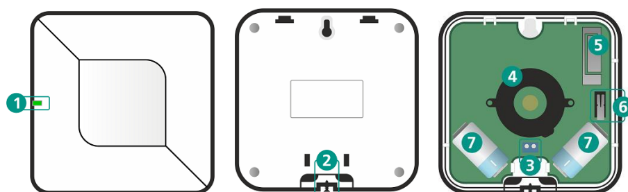
Рисунок 2.17 – Внешний вид сирены
